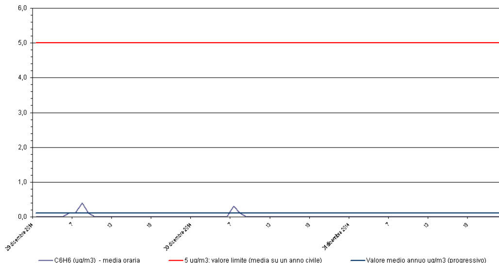
Benzene - C 6 H 6 Stazione di rilevamento di Sambruson, periodo: 29 dic 2014 - 31 dic 2014
