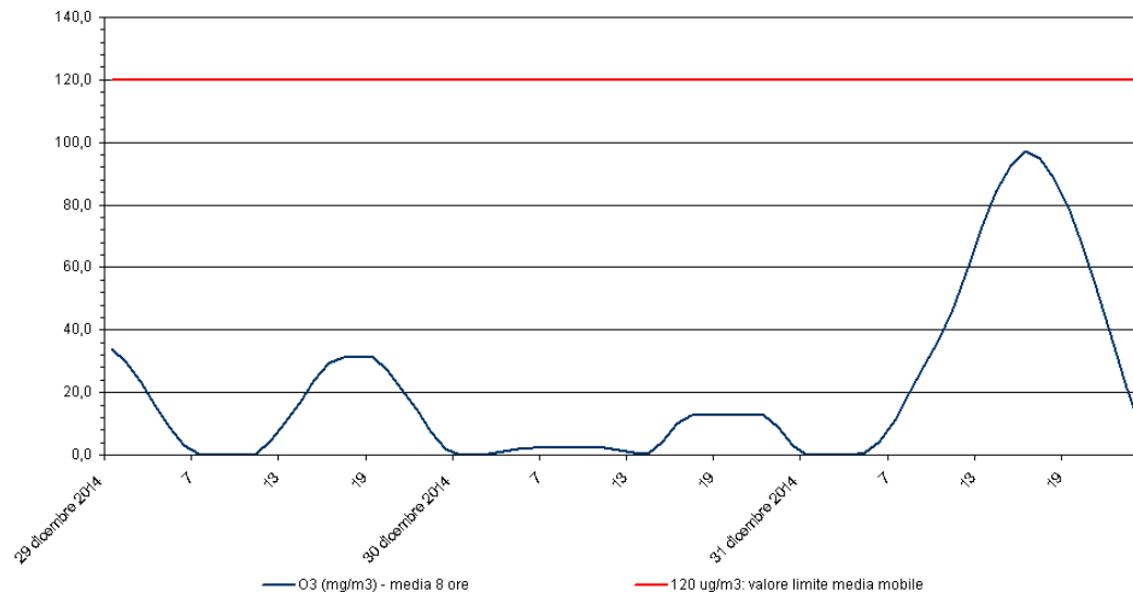
Ozono - O 3 Stazione di rilevamento di Sambruson, periodo: 29 dic 2014 - 31 dic 2014
