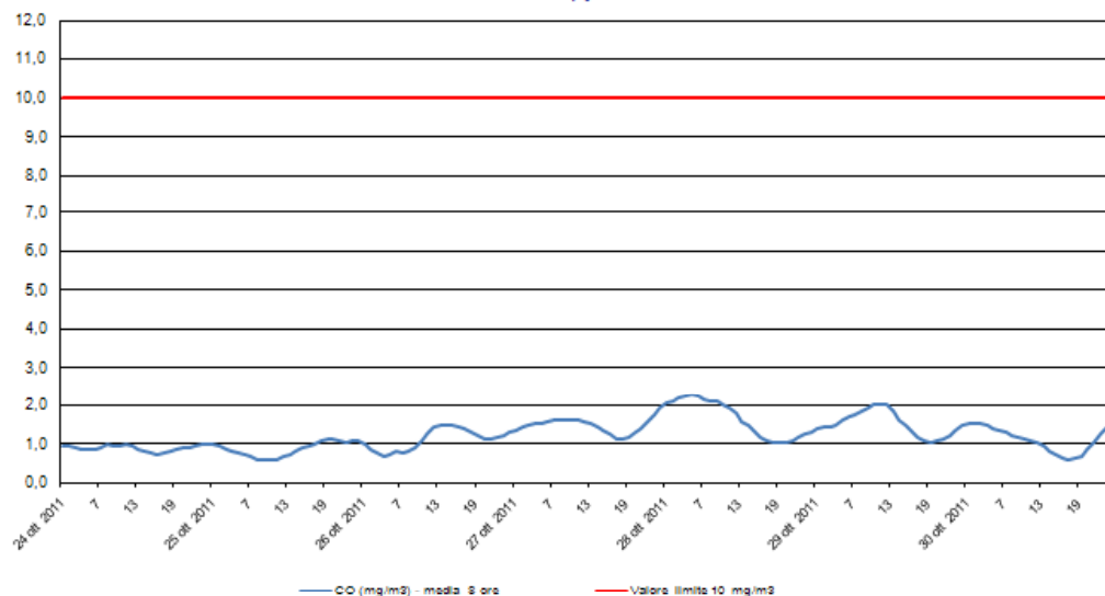
Monossido di Carbonio - CO Stazione di rilevamento di via B. Cairoli, periodo: 24 ott 2011 - 30 ott 2011
