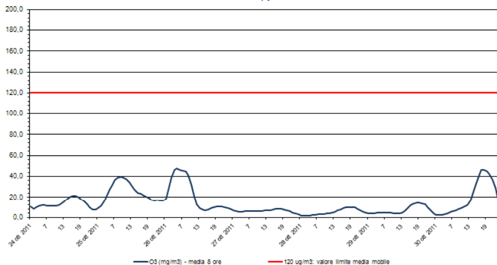
Ozono - O 3 Stazione di rilevamento di via B. Cairoli, periodo: 24 ott 2011 - 30 ott 2011
