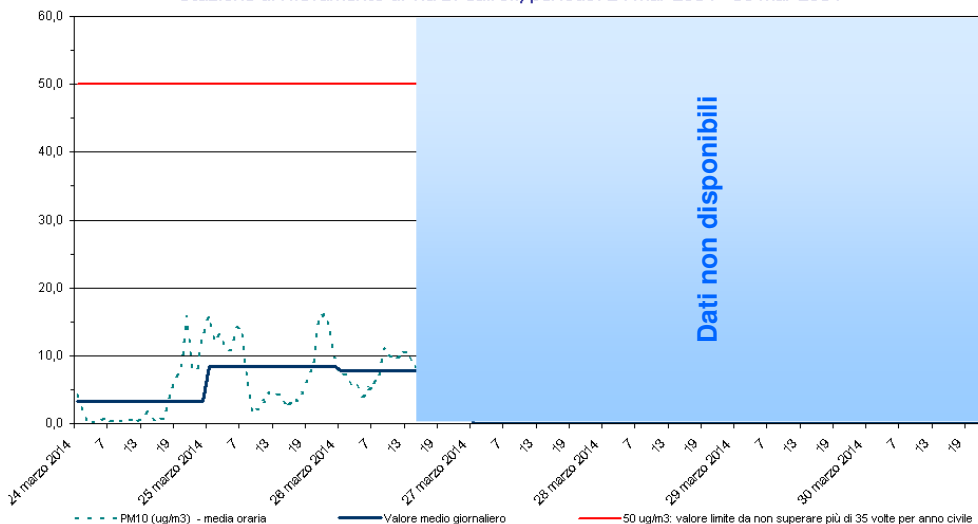
PM10 Stazione di rilevamento di via B. Cairoli, periodo: 24 mar 2014 - 30 mar 2014
