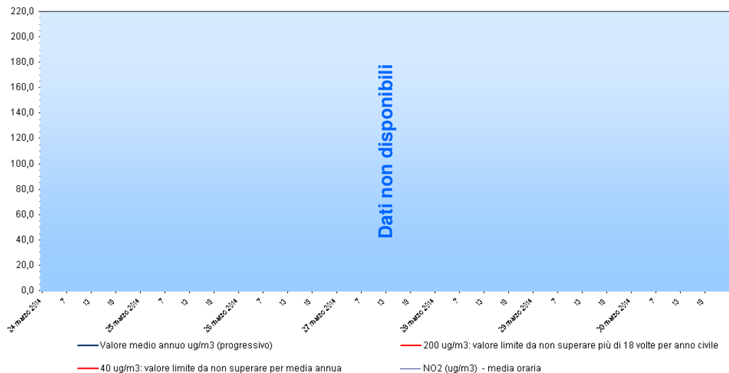
Biossido di azoto - NO 2 Stazione di rilevamento di Sambruson, periodo: 24 mar 2014 - 30 mar 2014
