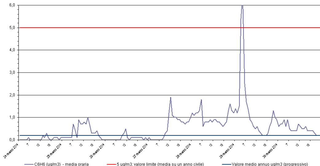
Benzene - C 6 H 6 Stazione di rilevamento di Sambruson, periodo: 24 mar 2014 - 30 mar 2014
