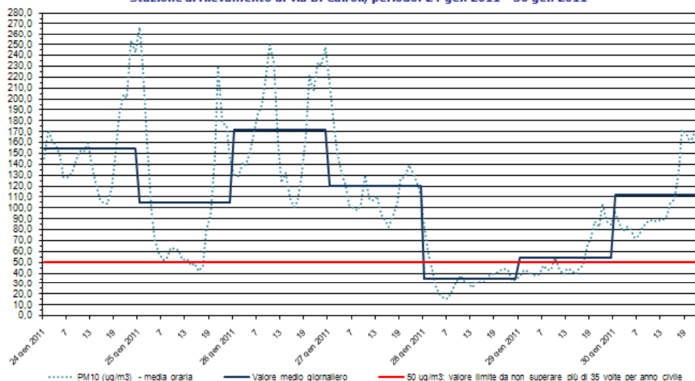
PM 10 Stazione di rilevamento di via B. Cairoli, periodo: 24 gen 2011 - 30 gen 2011
