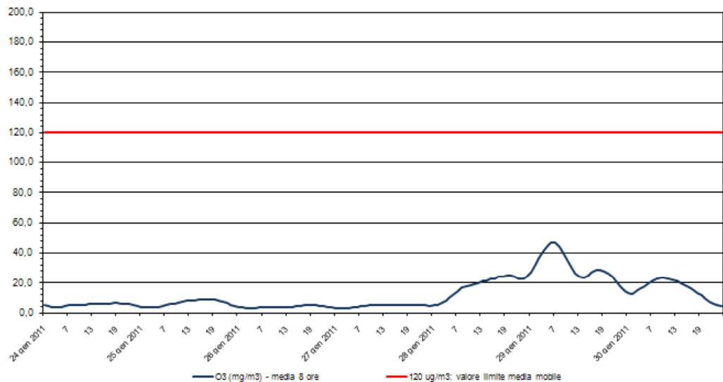
Ozono - O3 Stazione di rilevamento di via B. Cairoli, periodo: 24 gen 2011 - 30 gen 2011
