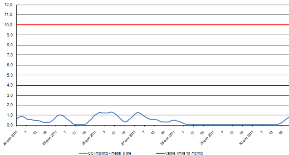
Monossido di Carbonio - CO Stazione di rilevamento di via B. Cairoli, periodo: 24 gen 2011 - 30 gen 2011
