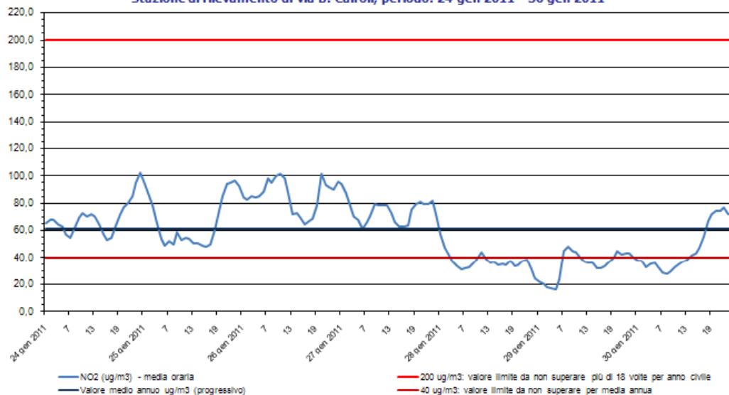
Biossido di azoto - NO 2 Stazione di rilevamento di via B. Cairoli, periodo: 24 gen 2011 - 30 gen 2011
