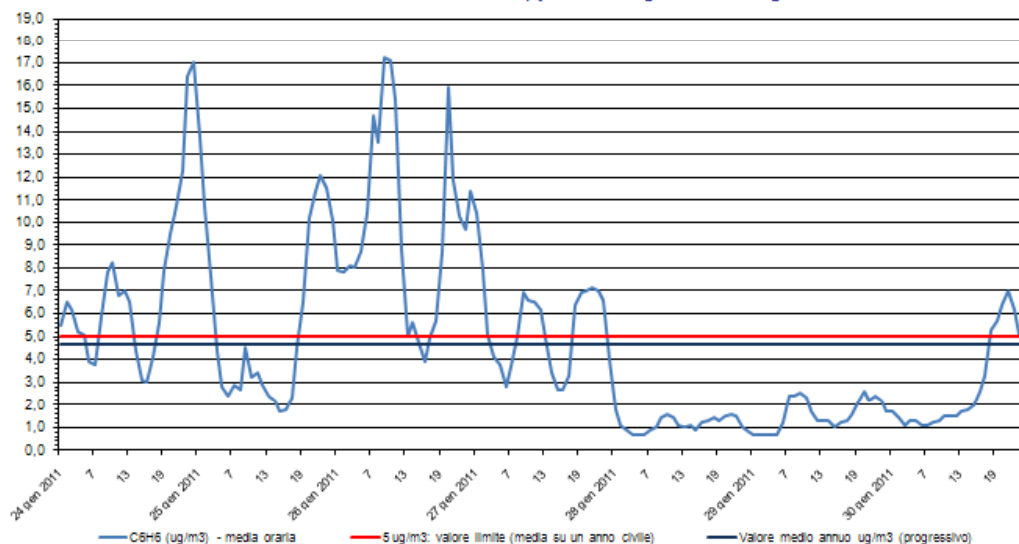
Benzene - C 6 H 6 Stazione di rilevamento di via B. Cairoli, periodo: 24 gen 2011 - 30 gen 2011
