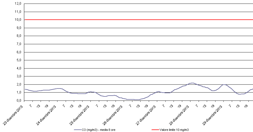
Monossido di Carbonio - CO Stazione di rilevamento di via B. Cairoli, periodo: 23 dic 2013 - 29 dic 2013
