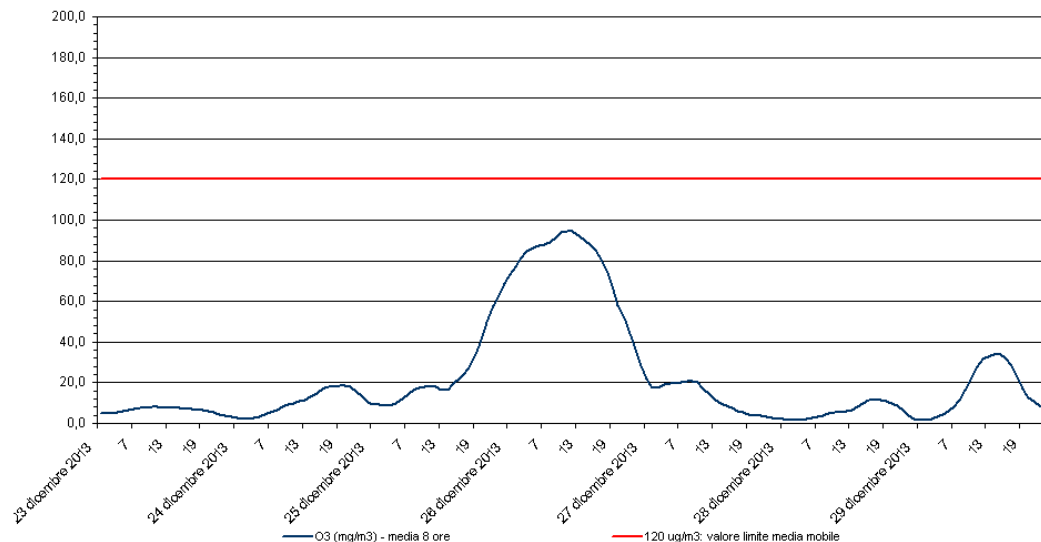
Ozono - O 3 Stazione di rilevamento di via B. Cairoli, periodo: 23 dic 2013 - 29 dic 2013
