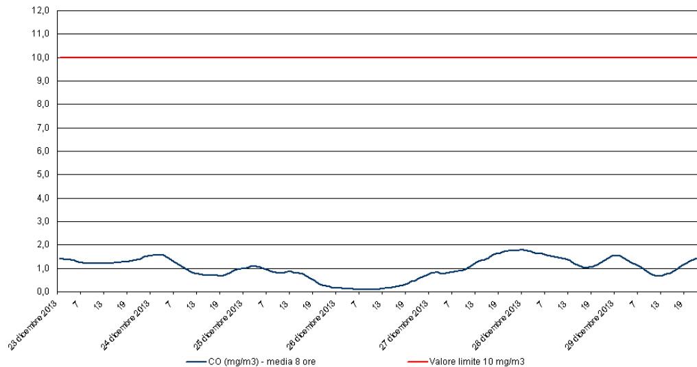
Monossido di Carbonio - CO Stazione di rilevamento di Sambruson, periodo: 23 dic 2013 - 29 dic 2013
