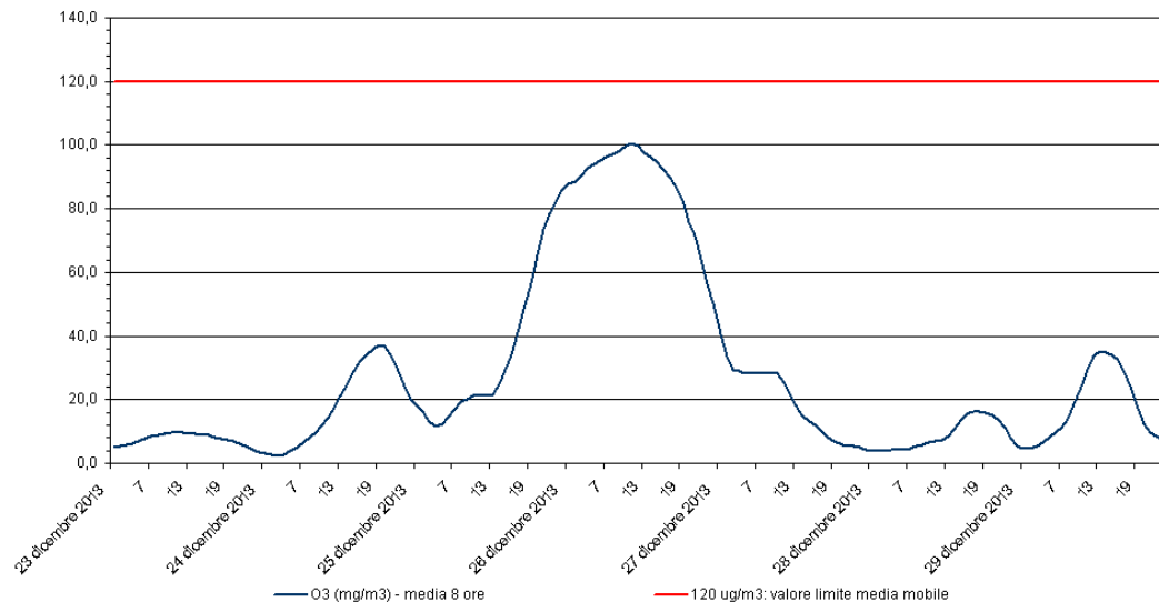
Ozono - O 3 Stazione di rilevamento di Sambruson, periodo: 23 dic 2013 - 29 dic 2013
