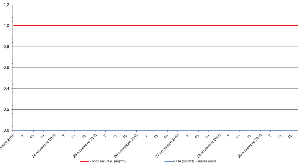
Metano - CH 4 Stazione di rilevamento di via B. Cairoli, periodo: 23 nov 2015 - 29 nov 2015
