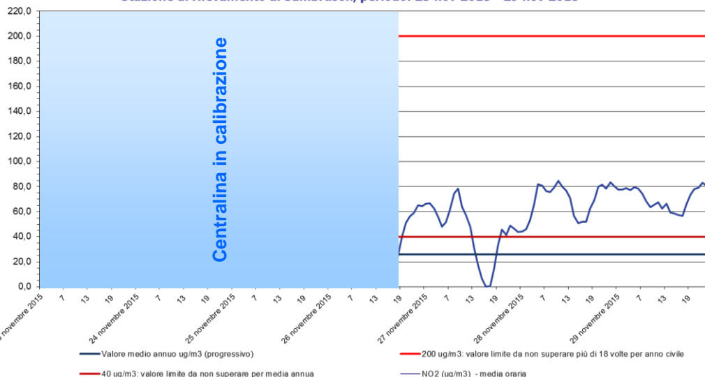
Biossido di azoto - NO 2 Stazione di rilevamento di Sambruson, periodo: 23 nov 2015 - 29 nov 2015
