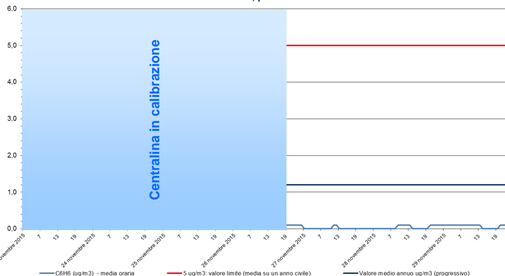
Benzene - C 6 H 6 Stazione di rilevamento di Sambruson, periodo: 23 nov 2015 - 29 nov 2015
