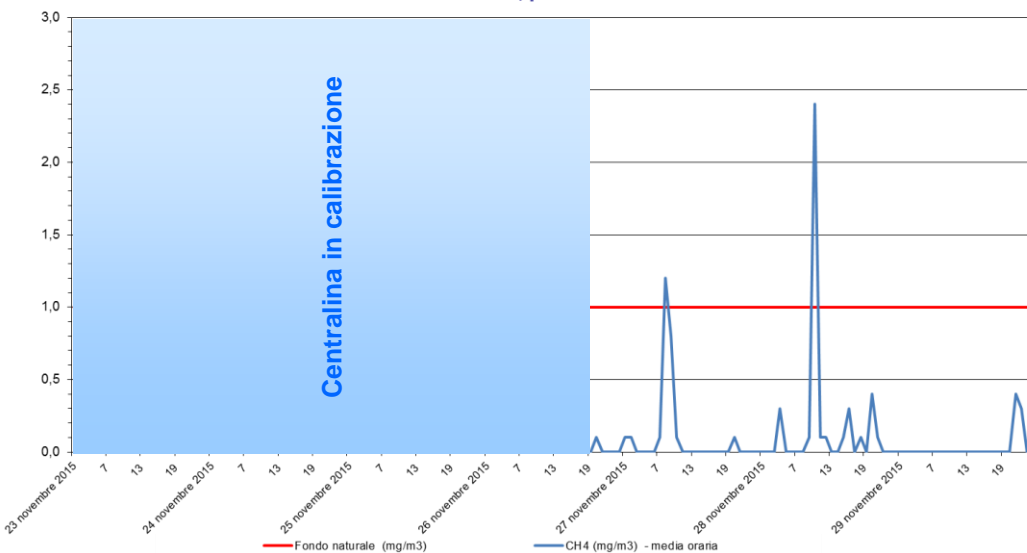
Metano - CH 4 Stazione di rilevamento di Sambruson, periodo: 23 nov 2015 - 29 nov 2015
