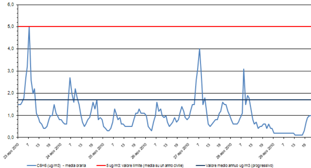
Benzene - C 6 H 6 Stazione di rilevamento di via B. Cairoli, periodo: : 23 ago 2010 - 29 ago 2010
