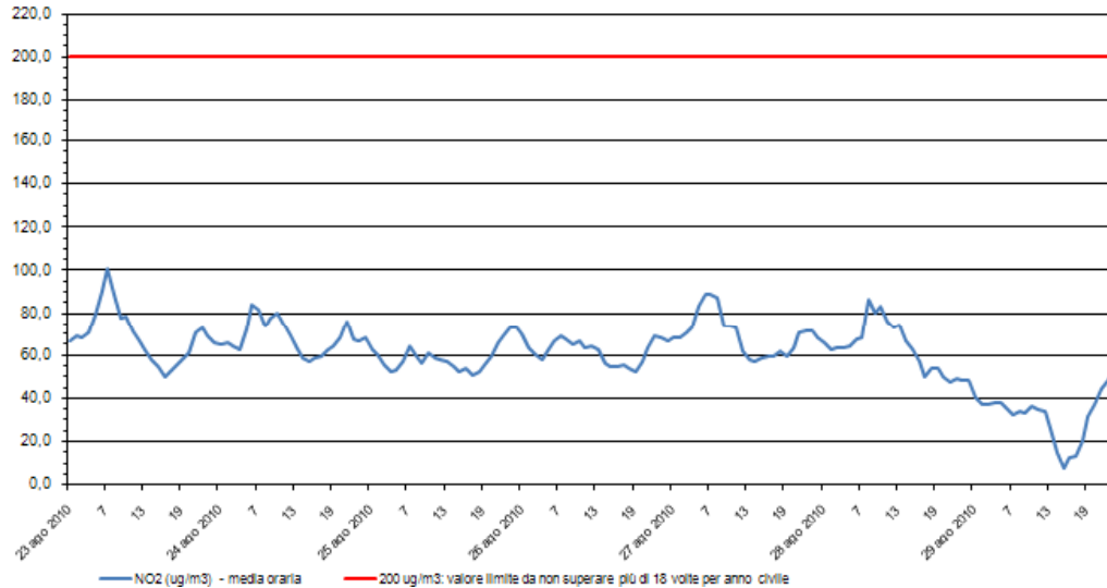
Biossido di azoto - NO 2 Stazione di rilevamento di via B. Cairoli, periodo: : 23 ago 2010 - 29 ago 2010
