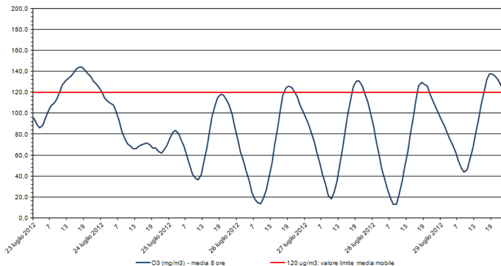
Ozono - O 3 Stazione di rilevamento di via B. Cairoli, periodo: 23 lug 2012- 29 lug 2012
