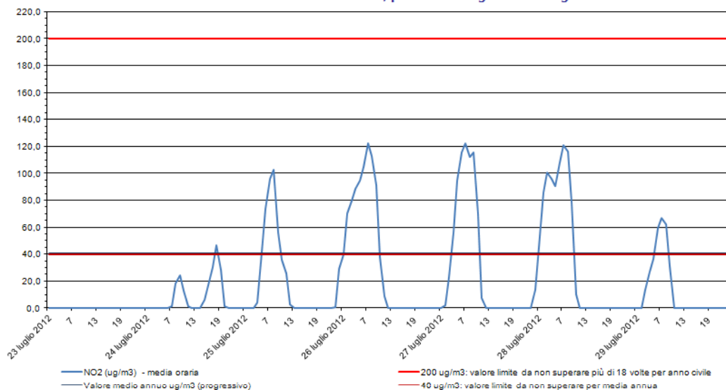
Biossido di azoto - NO 2 Stazione di rilevamento di via B. Cairoli, periodo: 23 lug 2012- 29 lug 2012
