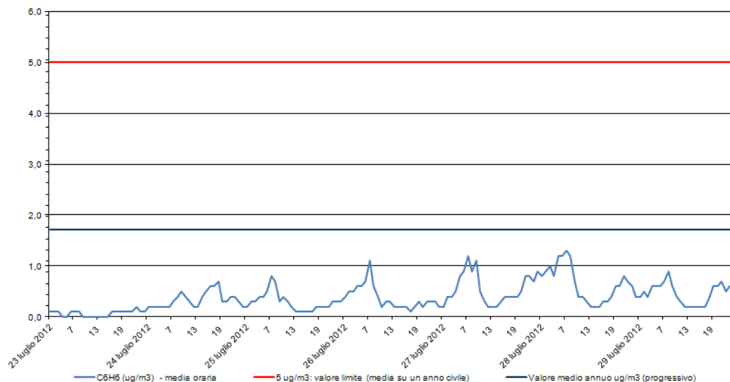
Benzene - C 6 H 6 Stazione di rilevamento di via B. Cairoli, periodo: 23 lug 2012- 29 lug 2012
