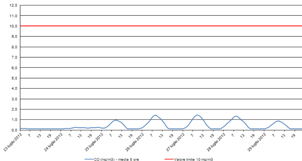
Monossido di Carbonio - CO Stazione di rilevamento di via B. Cairoli, periodo: 23 lug 2012- 29 lug 2012
