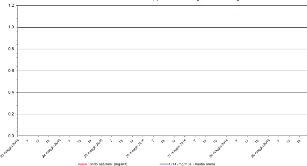
Metano - CH 4 Stazione di rilevamento di Sambruson, periodo: 23 mag 2016 - 29 mag 2016
