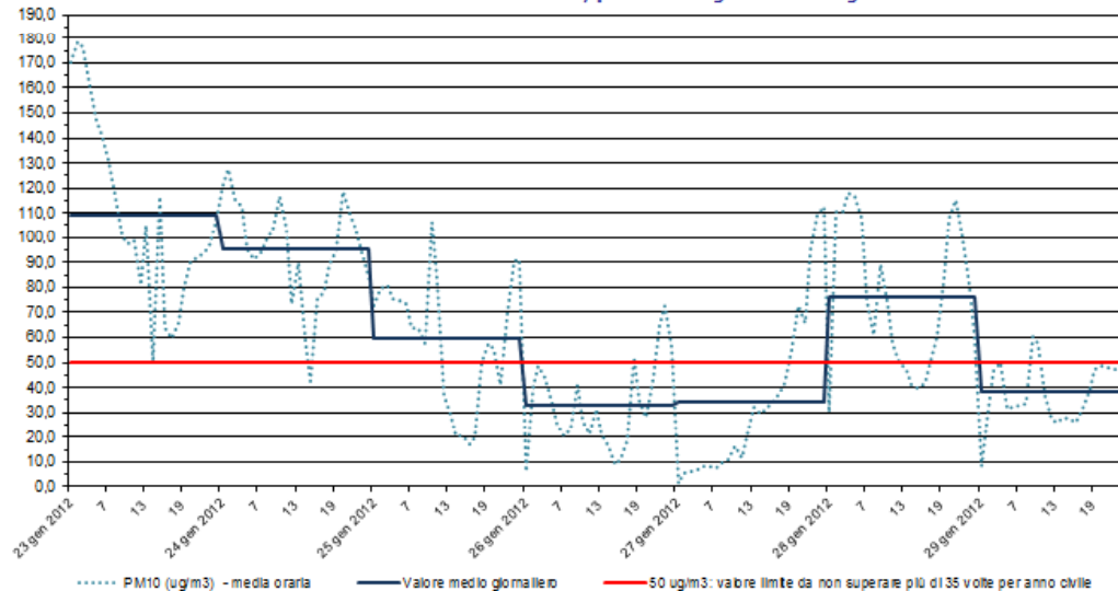
PM10 Stazione di rilevamento di via B. Cairoli, periodo: 23 gen 2012- 29 gen 2012
