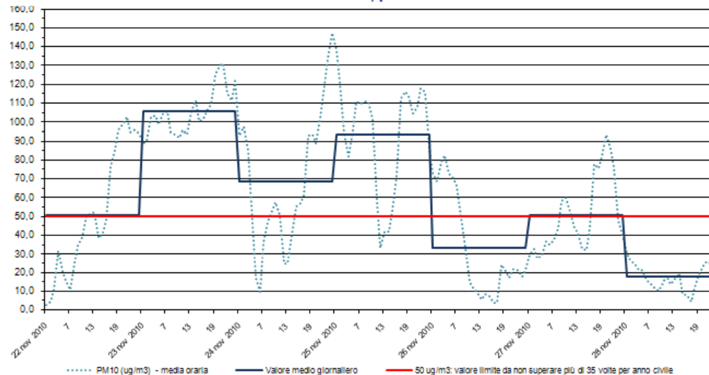
PM10 Stazione di rilevamento di via B. Cairoli, periodo: 22 nov 2010 - 28 nov 2010
