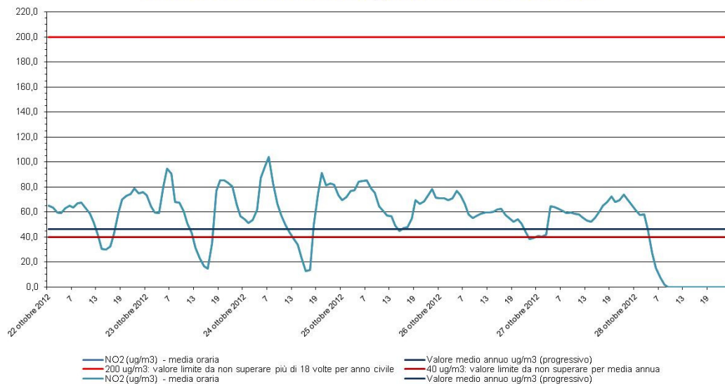
Biossido di azoto - NO 2 Stazione di rilevamento di Sambruson, periodo: 22 ott 2012 - 28 ott 2012
