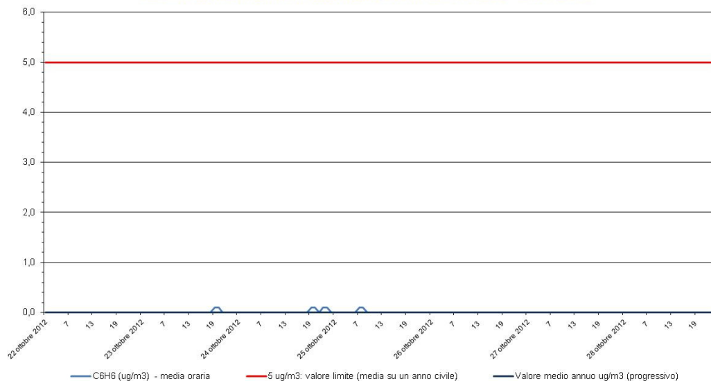
Benzene - C 6 H 6 Stazione di rilevamento di Sambruson, periodo: 22 ott 2012 - 28 ott 2012
