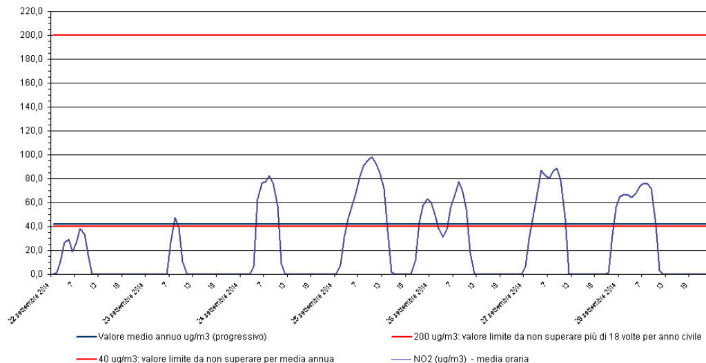
Biossido di azoto - NO 2 Stazione di rilevamento di Sambruson, periodo: 22 set 2014 - 28 set 2014
