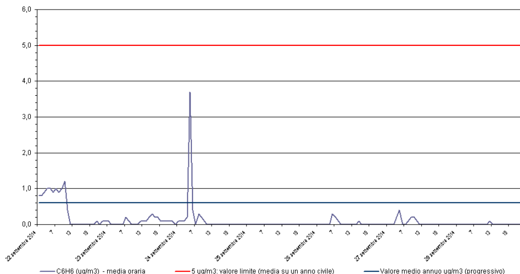
Benzene - C 6 H 6 Stazione di rilevamento di Sambruson, periodo: 22 set 2014 - 28 set 2014
