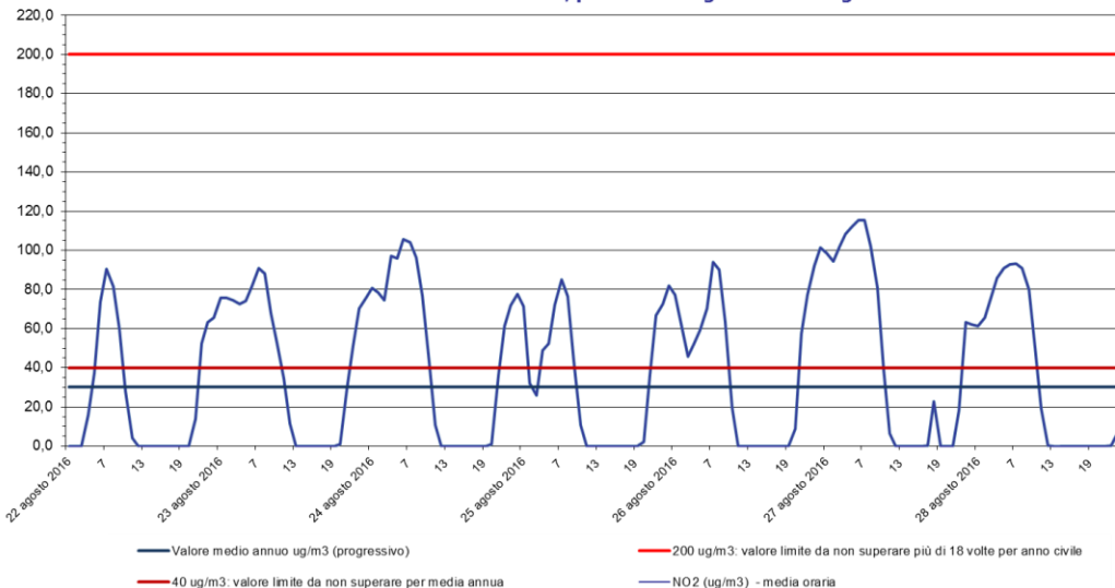
Biossido di azoto - NO 2 Stazione di rilevamento di Sambruson, periodo: 22 ago 2016 - 28 ago 2016
