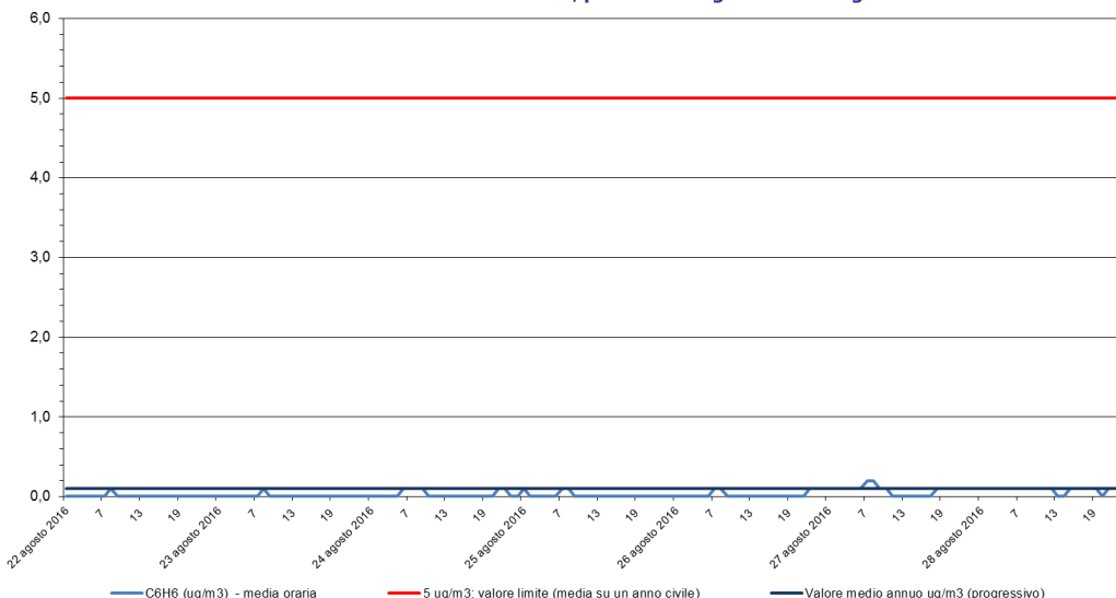
Benzene - C 6 H 6 Stazione di rilevamento di Sambruson, periodo: 22 ago 2016 - 28 ago 2016
