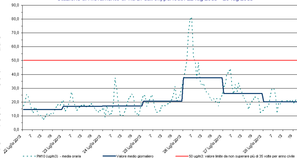
PM10 Stazione di rilevamento di via B. Cairoli, periodo: 22 lug 2013 - 28 lug 2013
