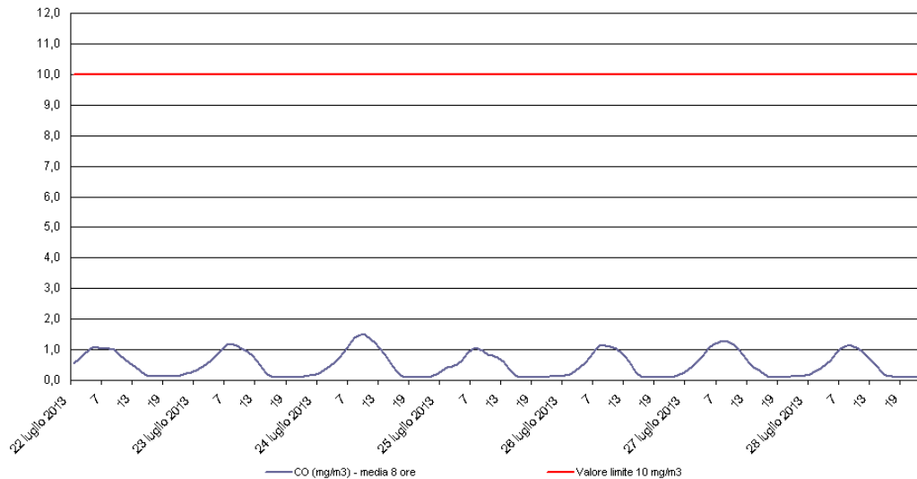
Monossido di Carbonio - CO Stazione di rilevamento di via B. Cairoli, periodo: 22 lug 2013 - 28 lug 2013
