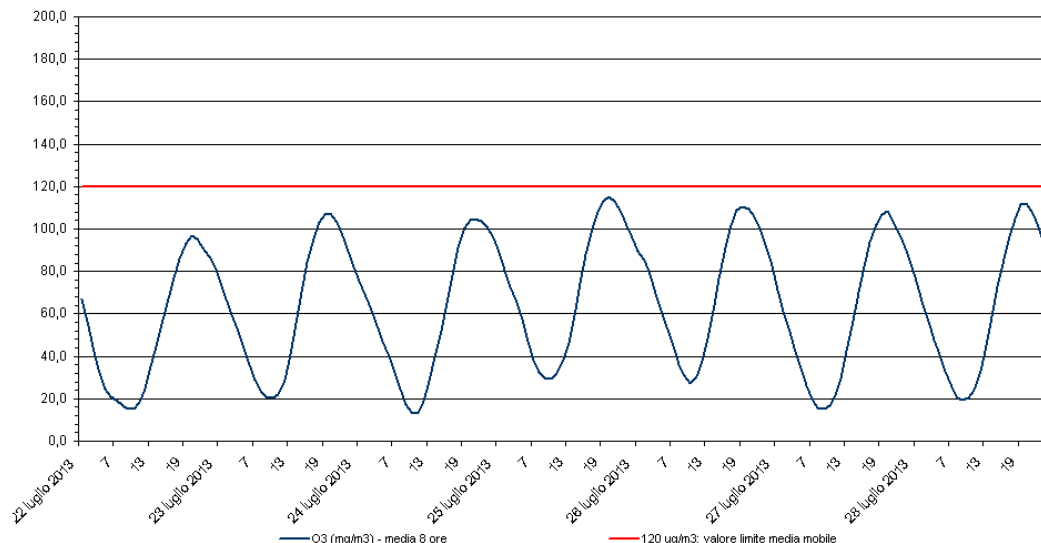
Ozono - O 3 Stazione di rilevamento di via B. Cairoli, periodo: 22 lug 2013 - 28 lug 2013
