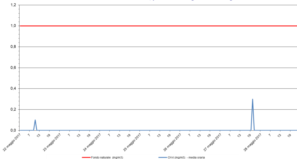
Metano - CH 4 Stazione di rilevamento di Sambruson, periodo: 22 mag 2017 - 28 mag 2017
