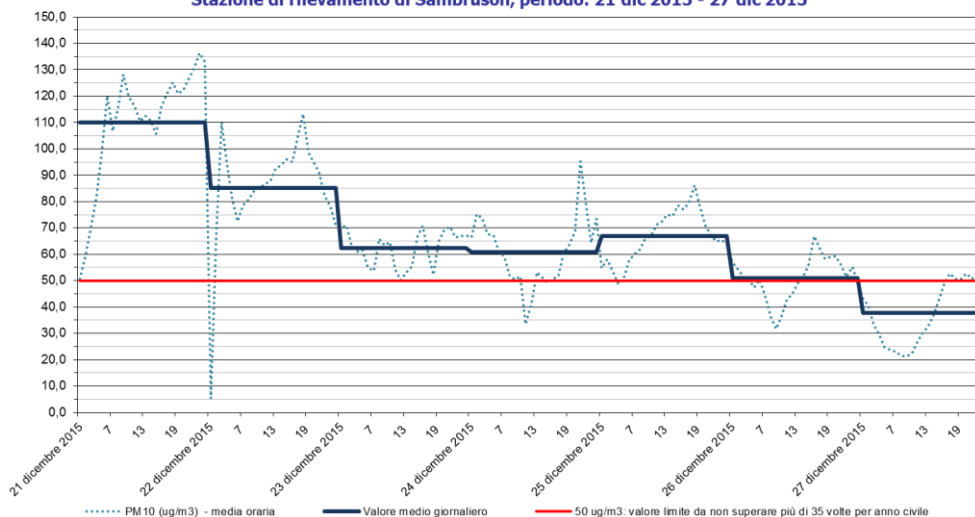
PM10 Stazione di rilevamento di Sambruson, periodo: 21 dic 2015 - 27 dic 2015
