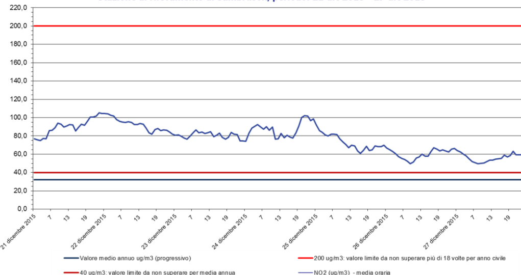
Biossido di azoto - NO 2 Stazione di rilevamento di Sambruson, periodo: 21 dic 2015 - 27 dic 2015
