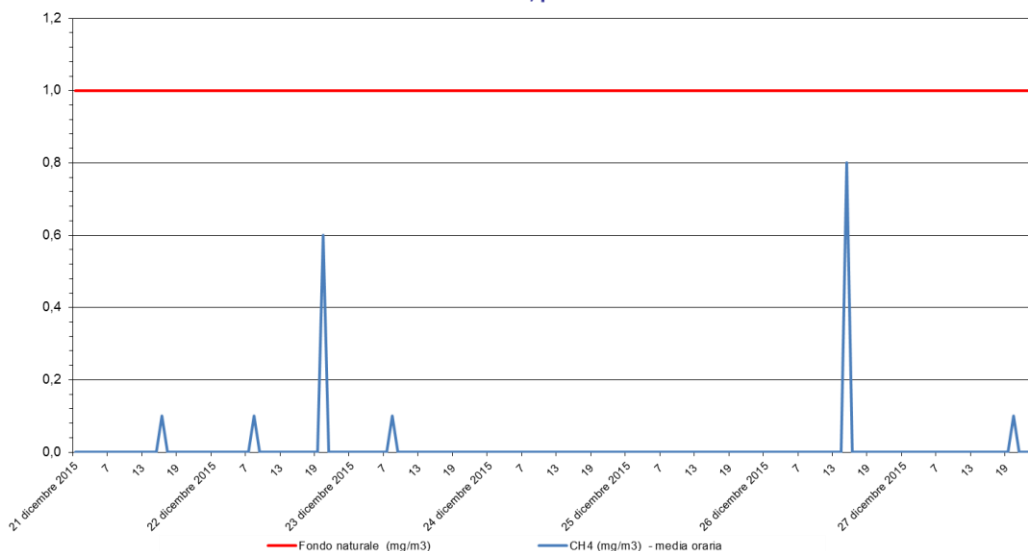
Metano - CH 4 Stazione di rilevamento di Sambruson, periodo: 21 dic 2015 - 27 dic 2015
