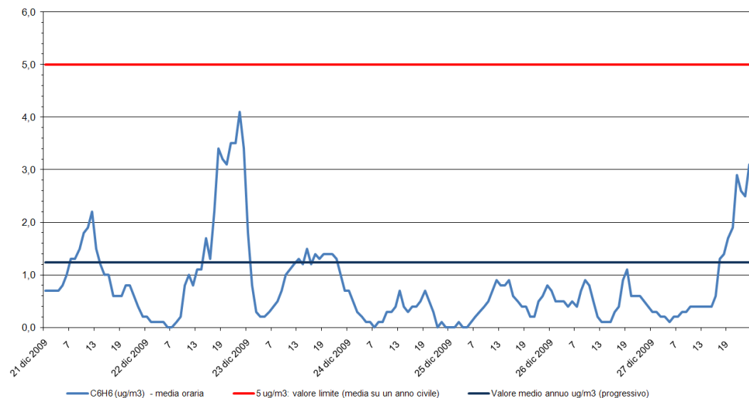
Benzene - C 6 H 6 Stazione di rilevamento di via F.lli Bandiera, periodo: 21 dic 2009 - 27 dic 2009
