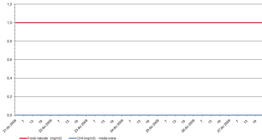
Metano - CH 4 Stazione di rilevamento di via F.lli Bandiera, periodo: 21 dic 2009- 27 dic 2009
