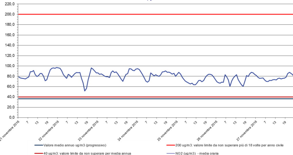
Biossido di azoto - NO 2 Stazione di rilevamento di Sambruson, periodo: 21 nov 2016 - 27 nov 2016
