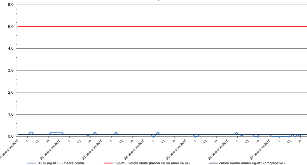
Benzene - C 6 H 6 Stazione di rilevamento di Sambruson, periodo: 21 nov 2016 - 27 nov 2016
