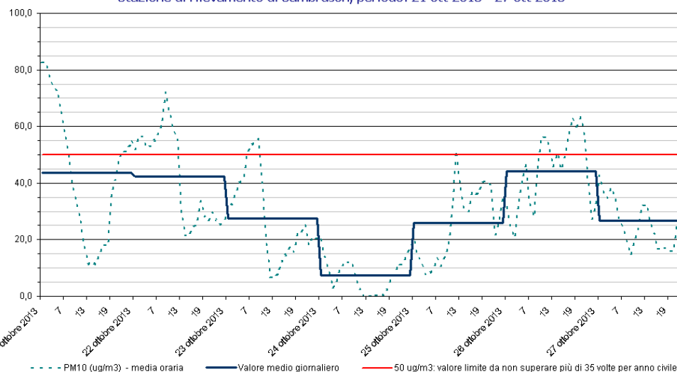
PM10 Stazione di rilevamento di Sambruson, periodo: 21 ott 2013 - 27 ott 2013
