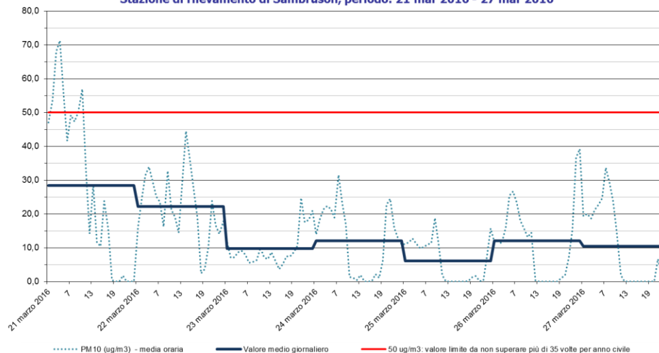
PM10 Stazione di rilevamento di Sambruson, periodo: 21 mar 2016 - 27 mar 2016
