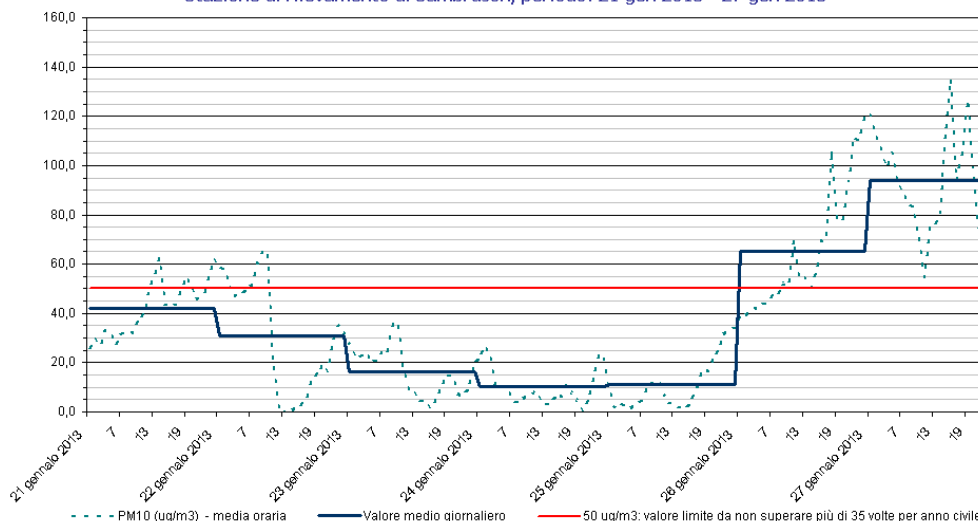
PM10 Stazione di rilevamento di Sambruson, periodo: 21 gen 2013 - 27 gen 2013
