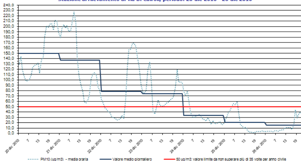
PM10 Stazione di rilevamento di via B. Cairoli, periodo: 20 dic 2010 - 26 dic 2010
