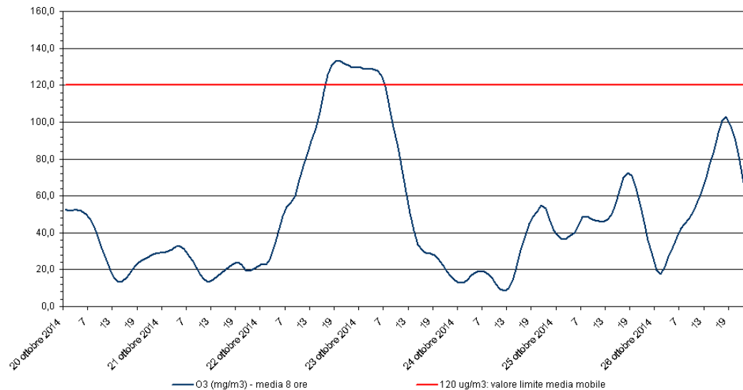
Ozono - O 3 Stazione di rilevamento di Sambruson, periodo: 20 ott 2014 - 26 ott 2014
