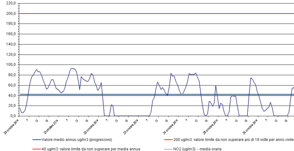
Biossido di azoto - NO 2 Stazione di rilevamento di Sambruson, periodo: 20 ott 2014 - 26 ott 2014
