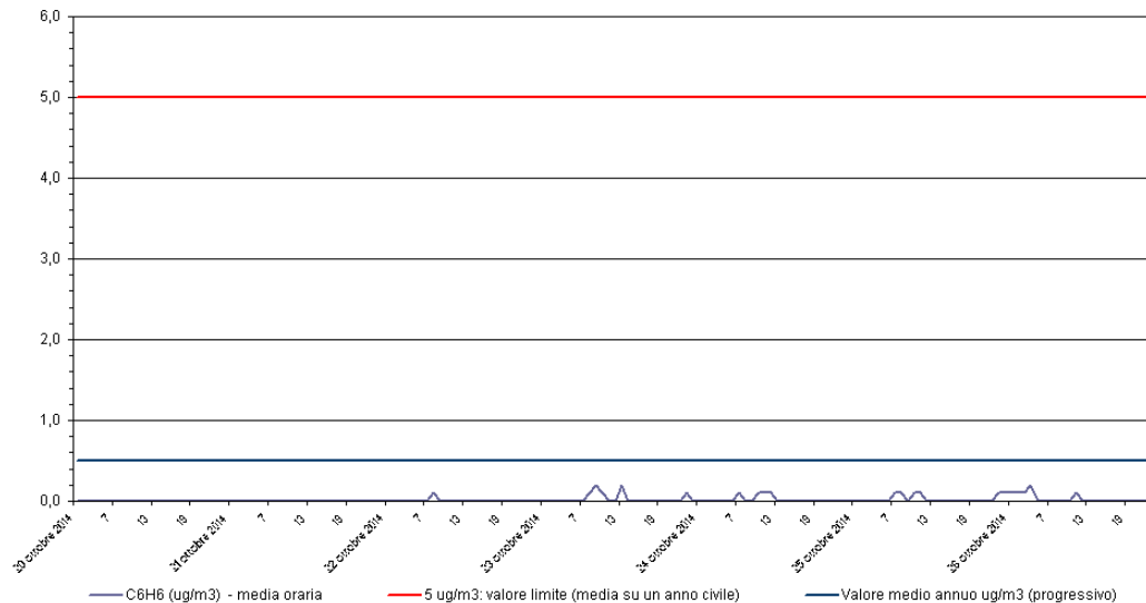
Benzene - C 6 H 6 Stazione di rilevamento di Sambruson, periodo: 20 ott 2014 - 26 ott 2014
