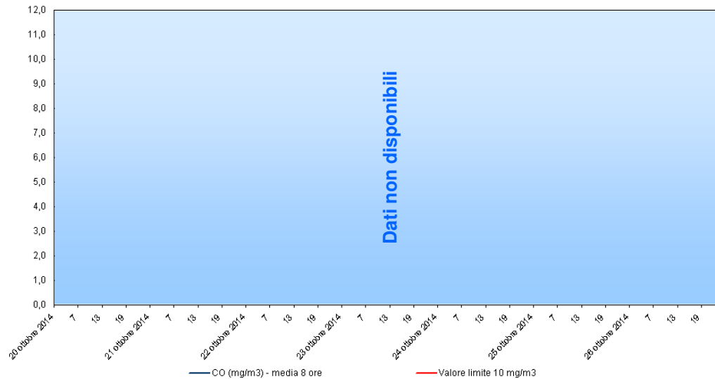
Monossido di Carbonio - CO Stazione di rilevamento di Sambruson, periodo: 20 ott 2014 - 26 ott 2014
