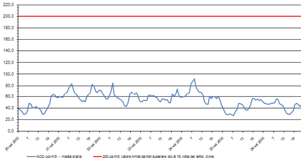
Biossido di azoto - NO 2 Stazione di rilevamento di via B. Cairoli, periodo: 20 set 2010 - 26 set 2010
