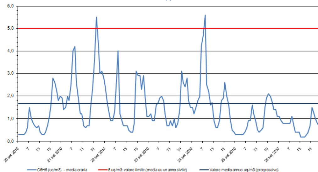
Benzene - C 6 H 6 Stazione di rilevamento di via B. Cairoli, periodo: 20 set 2010 - 26 set 2010
