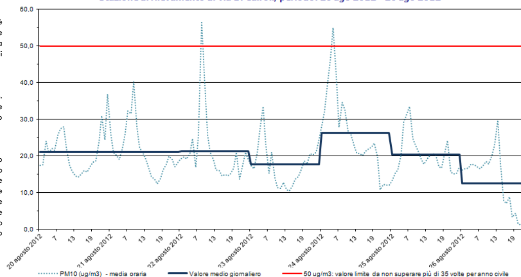
PM10 Stazione di rilevamento di via B. Cairoli, periodo: 20 ago 2012 - 26 ago 2012
