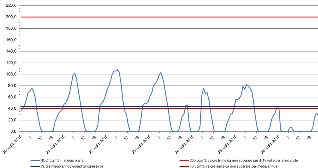
Biossido di azoto - NO 2 Stazione di rilevamento di via B. Cairoli, periodo: 20 lug 2015 - 26 lug 2015
