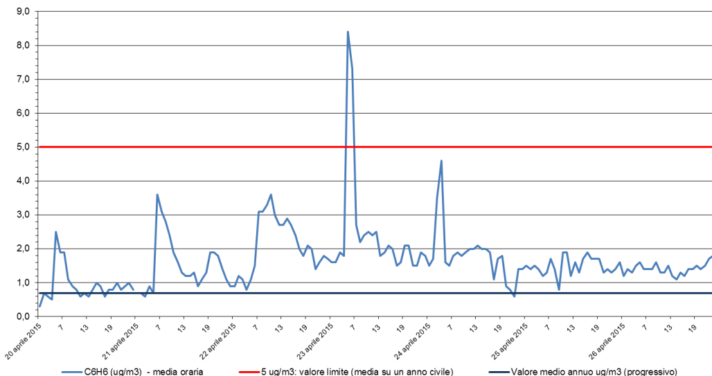
Benzene - C 6 H 6 Stazione di rilevamento di Sambruson, periodo: 20 apr 2015 - 26 apr 2015
