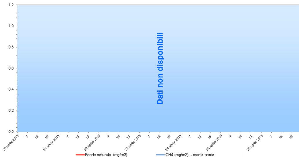
Metano - CH 4 Stazione di rilevamento di Sambruson, periodo: 20 apr 2015 - 26 apr 2015
