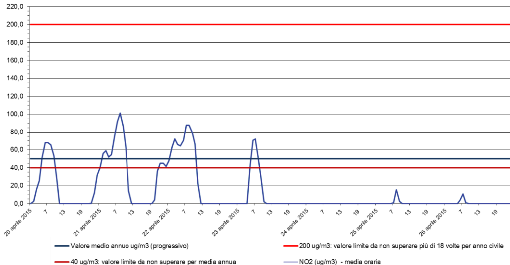
Biossido di azoto - NO 2 Stazione di rilevamento di Sambruson, periodo: 20 apr 2015 - 26 apr 2015
