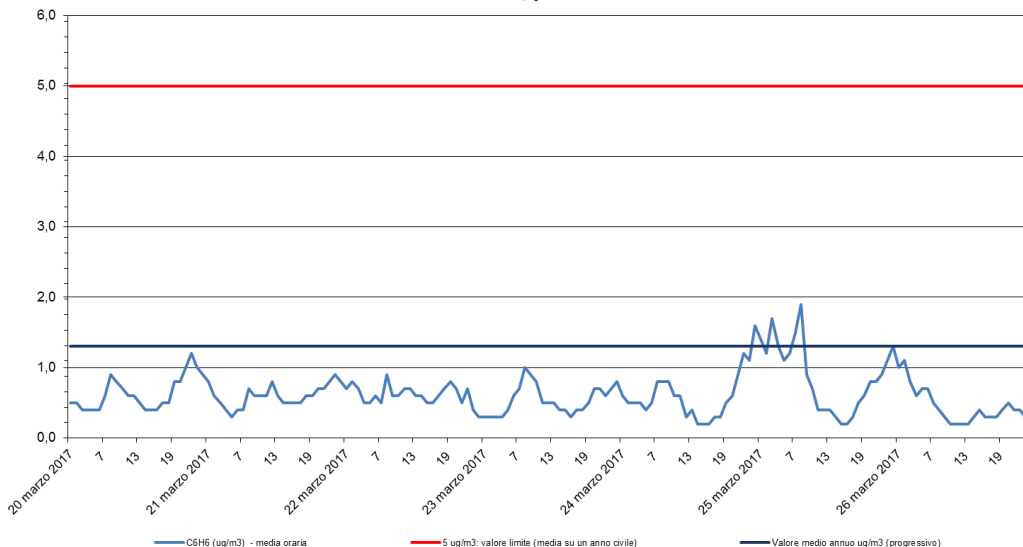
Benzene - C 6 H 6 Stazione di rilevamento di via B. Cairoli, periodo: 20 mar 2017 - 26 mar 2017
