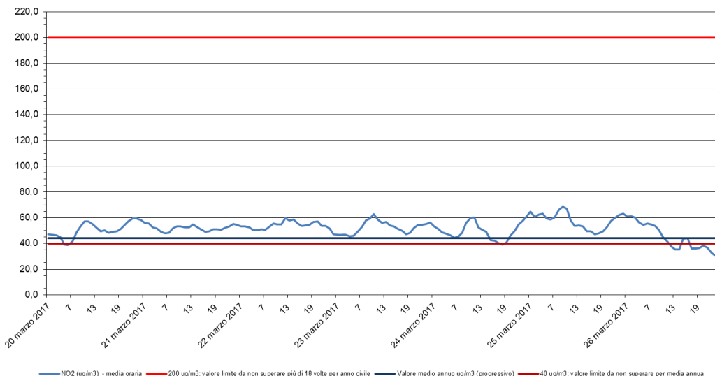
Biossido di azoto - NO 2 Stazione di rilevamento di via B. Cairoli, periodo: 20 mar 2017 - 26 mar 2017
