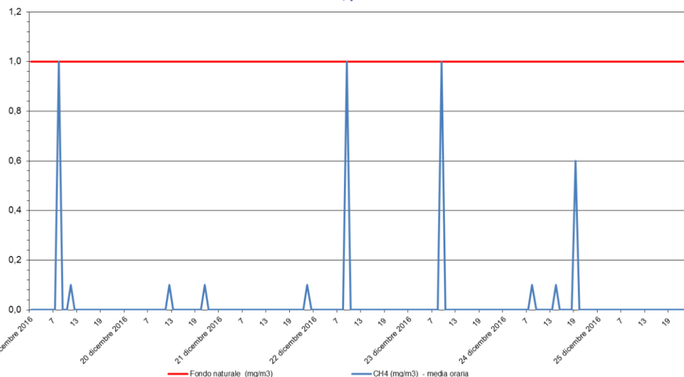
Metano - CH 4 Stazione di rilevamento di Sambruson, periodo: 19 dic 2016 - 25 dic 2016
