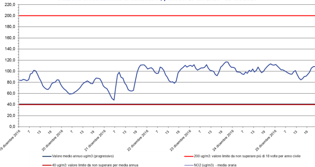
Biossido di azoto - NO 2 Stazione di rilevamento di Sambruson, periodo: 19 dic 2016 - 25 dic 2016
