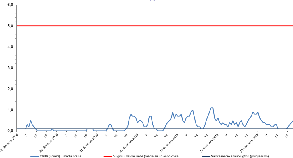
Benzene - C 6 H 6 Stazione di rilevamento di Sambruson, periodo: 19 dic 2016 - 25 dic 2016
