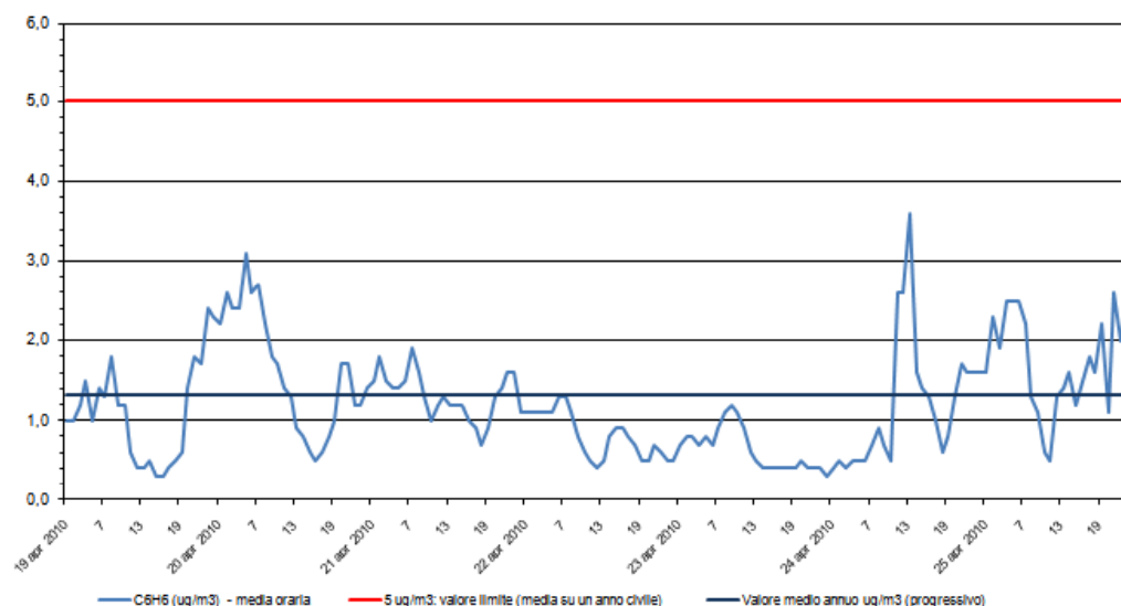
Benzene - C 6 H 6 Stazione di rilevamento di via F.lli Bandiera, periodo: 19 apr 2010 - 25 apr 2010
