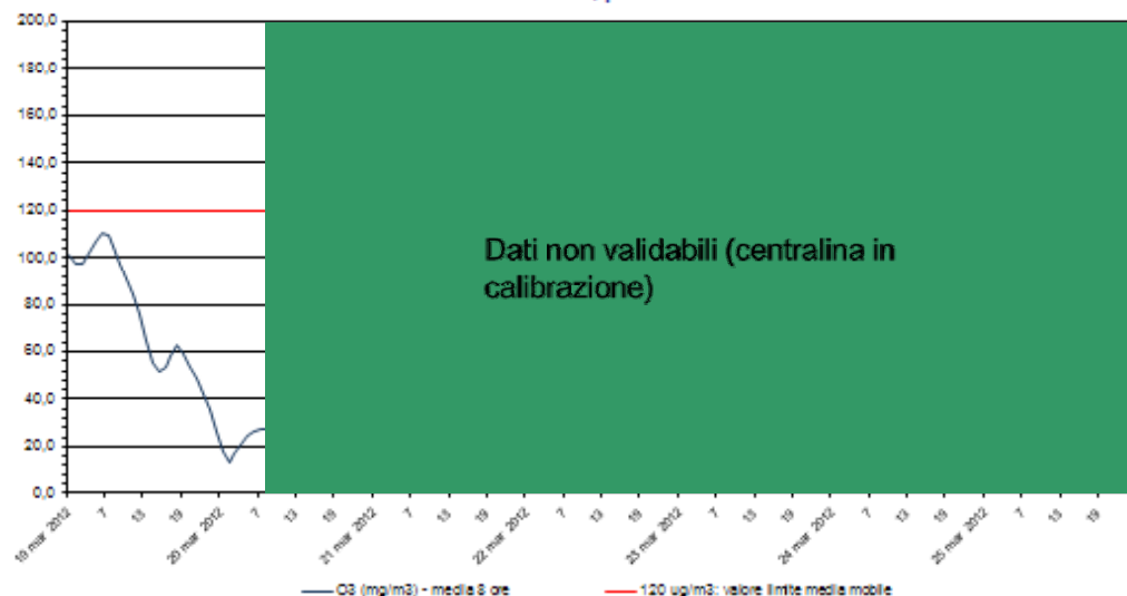
Ozono - O 3 Stazione di rilevamento di via B. Cairoli, periodo: 19 mar 2012- 25 mar 2012
