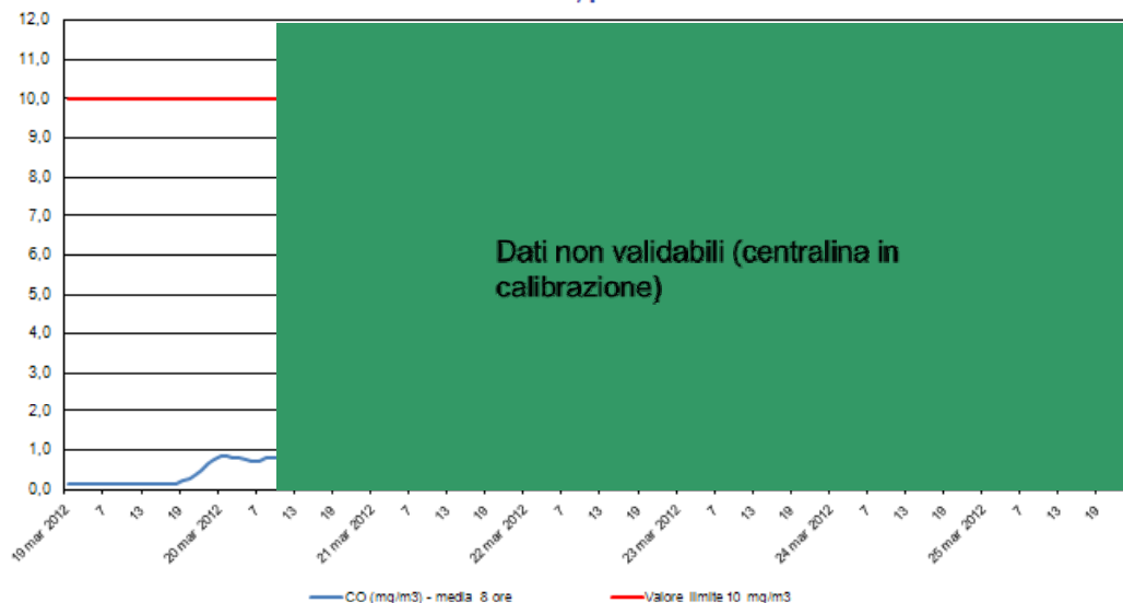
Monossido di Carbonio - CO Stazione di rilevamento di via B. Cairoli, periodo: 19 mar 2012- 25 mar 2012
