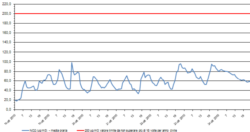
Biossido di azoto - NO 2 Stazione di rilevamento di via B. Cairoli, periodo: 18 ott 2010 - 24 ott 2010
