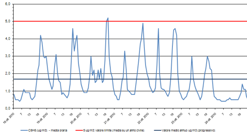
Benzene - C 6 H 6 Stazione di rilevamento di via B. Cairoli, periodo: 18 ott 2010 - 24 ott 2010
