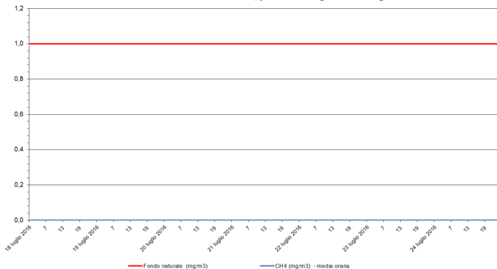
Metano - CH 4 Stazione di rilevamento di Sambruson, periodo: 18 lug 2016 - 24 lug 2016
