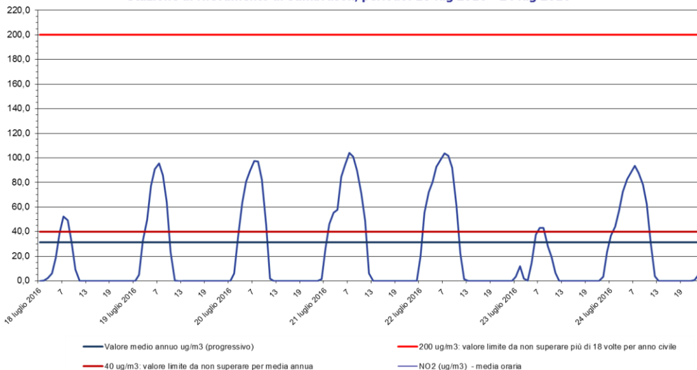
Biossido di azoto - NO 2 Stazione di rilevamento di Sambruson, periodo: 18 lug 2016 - 24 lug 2016
