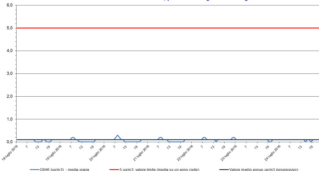
Benzene - C 6 H 6 Stazione di rilevamento di Sambruson, periodo: 18 lug 2016 - 24 lug 2016
