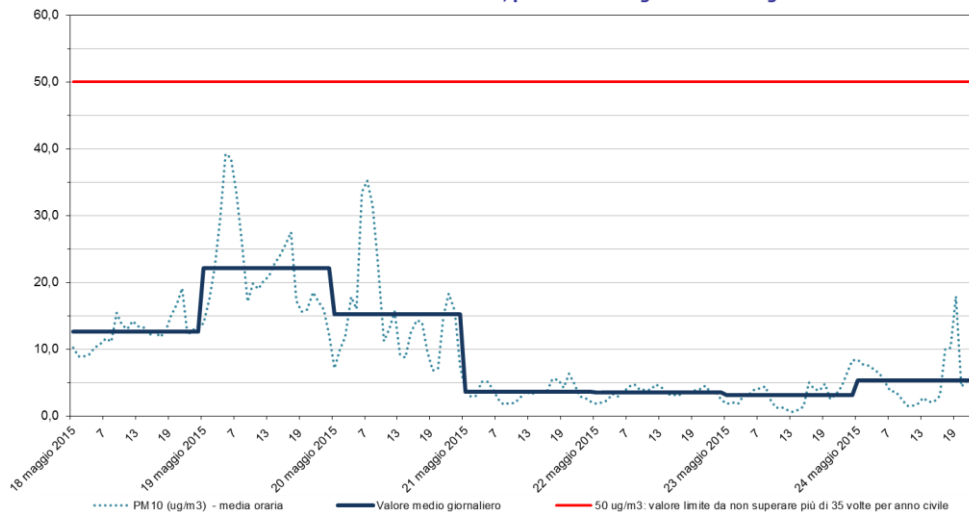
PM10 Stazione di rilevamento di via B. Cairoli, periodo: 18 mag 2015 - 24 mag 2015
