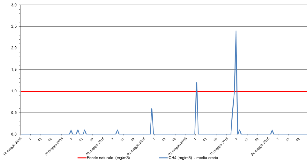
Metano - CH 4 Stazione di rilevamento di Sambruson, periodo: 18 mag 2015 - 24 mag 2015
