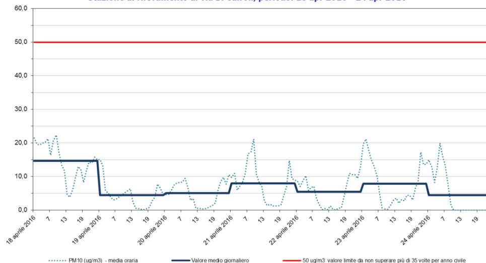
PM10 Stazione di rilevamento di via B. Cairoli, periodo: 18 apr 2016 - 24 apr 2016
