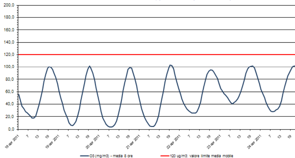
Ozono - O3 Stazione di rilevamento di via B. Cairoli, periodo: 18 apr 2011 - 24 apr 2011
