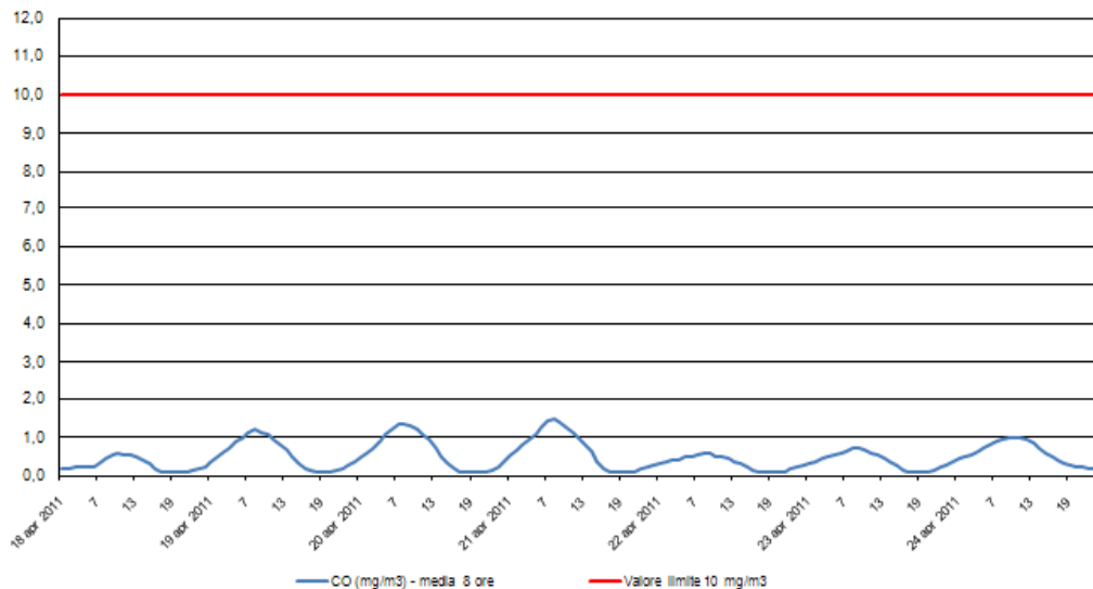
Monossido di Carbonio - CO Stazione di rilevamento di via B. Cairoli, periodo: 18 apr 2011 - 24 apr 2011
