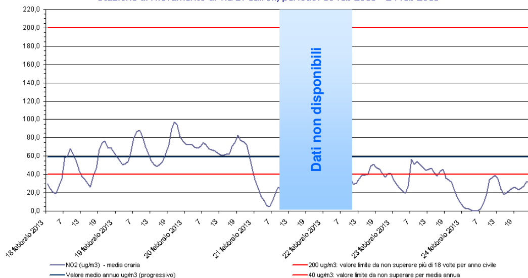
Biossido di azoto - NO 2 Stazione di rilevamento di via B. Cairolì, periodo: 18 feb 2013 - 24 feb 2013
