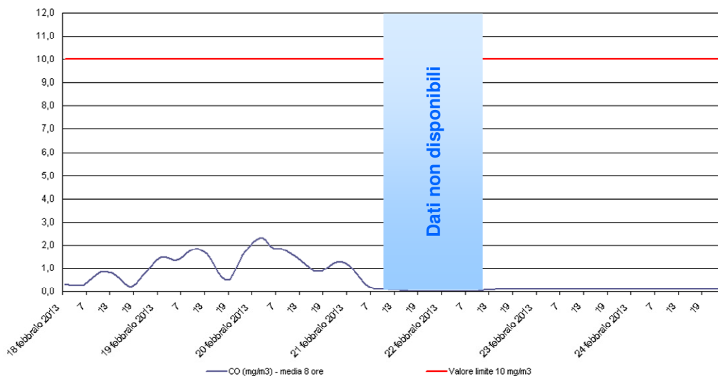
Monossido di Carbonio - CO Stazione di rilevamento di via B. Cairoli, periodo: 18 feb 2013 - 24 feb 2013
