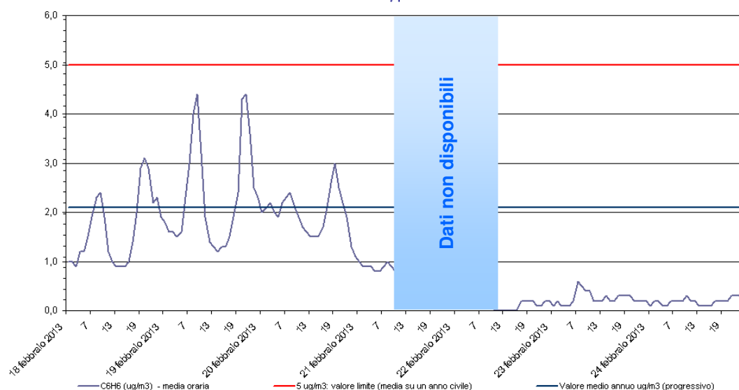
Benzene - C 6 H 6 Stazione di rilevamento di via B. Cairolì, periodo: 18 feb 2013 - 24 feb 2013
