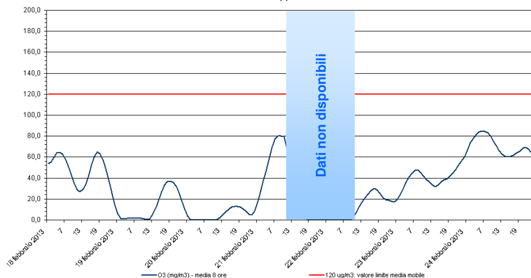
Ozono - O 3 Stazione di rilevamento di via B. Cairoli, periodo: 18 feb 2013 - 24 feb 2013
