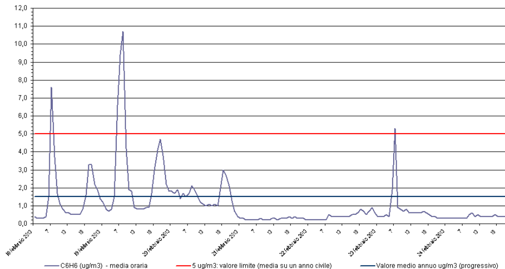
Benzene - C 6 H 6 Stazione di rilevamento di Sambruson, periodo: 18 feb 2013 - 24 feb 2013
