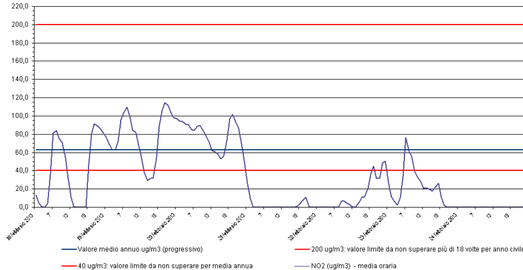
Biossido di azoto - NO 2 Stazione di rilevamento di Sambruson, periodo: 18 feb 2013 - 24 feb 2013
