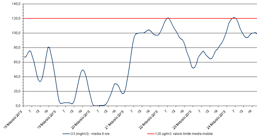
Ozono - O 3 Stazione di rilevamento di Sambruson, periodo: 18 feb 2013 - 24 feb 2013
