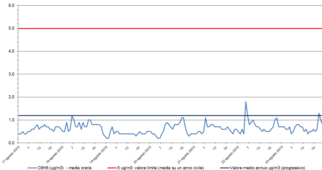
Benzene - C 6 H 6 Stazione di rilevamento di Sambruson, periodo: 17 ago 2015 - 23 ago 2015
