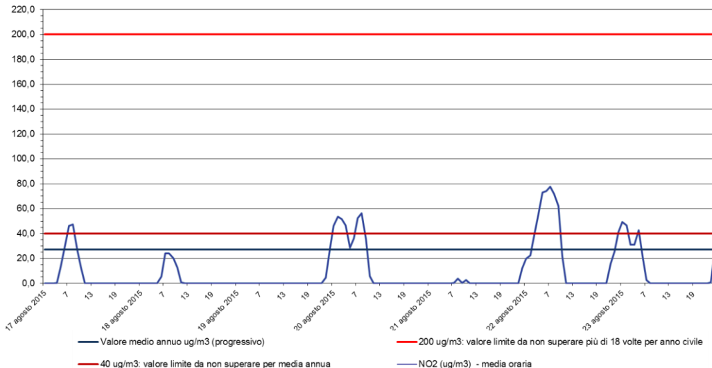
Biossido di azoto - NO 2 Stazione di rilevamento di Sambruson, periodo: 17 ago 2015 - 23 ago 2015
