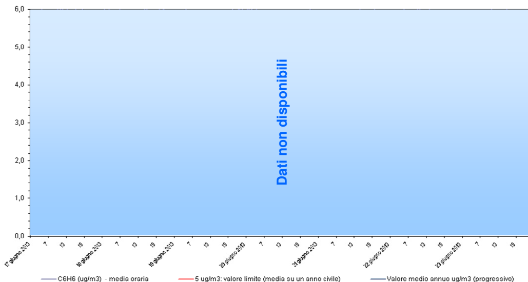
Benzene - C 6 H 6 Stazione di rilevamento di Sambruson, periodo: 17 giu 2013 - 23 giu 2013
