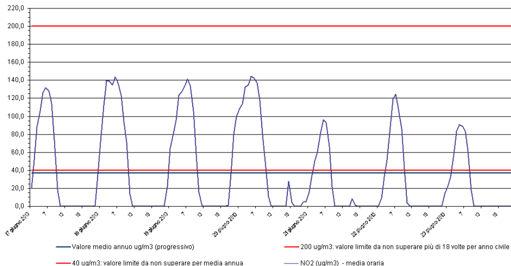
Biossido di azoto - NO 2 Stazione di rilevamento di Sambruson, periodo: 17 giu 2013 - 23 giu 2013
