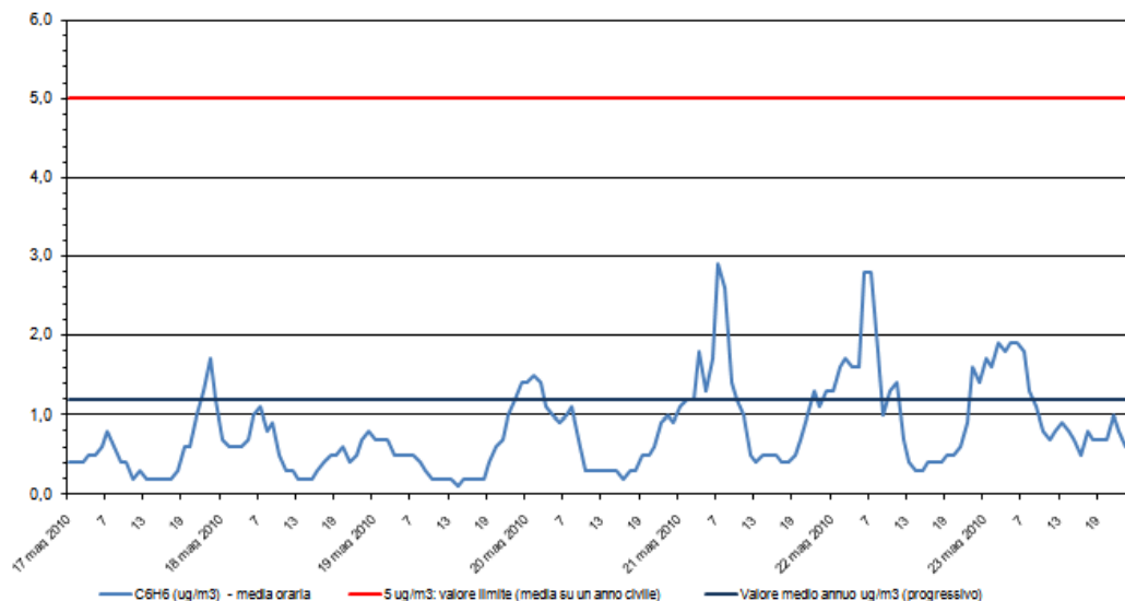
Benzene - C 6 H 6 Stazione di rilevamento di via F.lli Bandiera, periodo: 17 mag 2010 - 23 mag 2010
