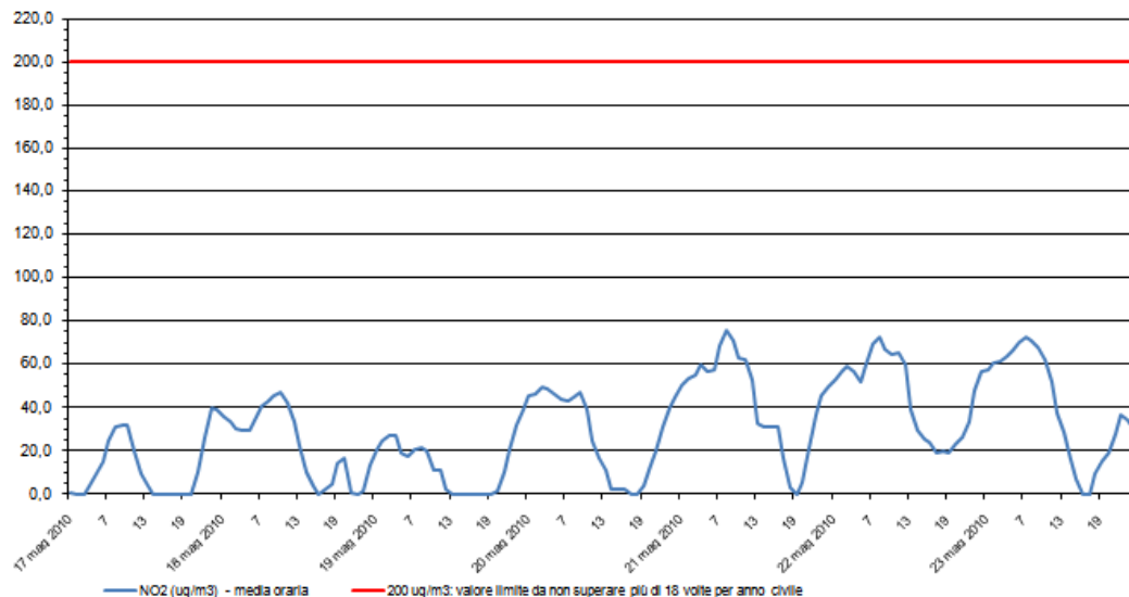
Biossido di azoto - NO 2 Stazione di rilevamento di via F.lli Bandiera, periodo: 17 mag 2010 - 23 mag 2010
