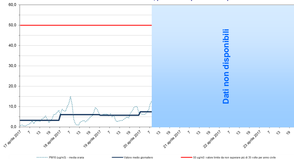
PM10 Stazione di rilevamento di via B. Cairoli, periodo: 17 apr 2017 - 23 apr 2017
